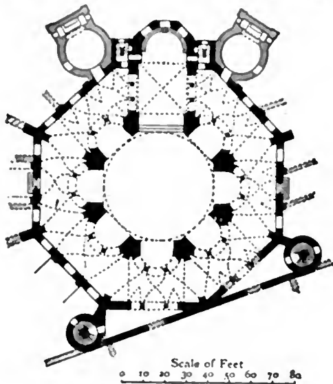
FIG. 30.—Plan of S. Vitale, Ravenna.
