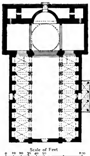
FIG. 39.—Plan of S. Nicola at Bari.
