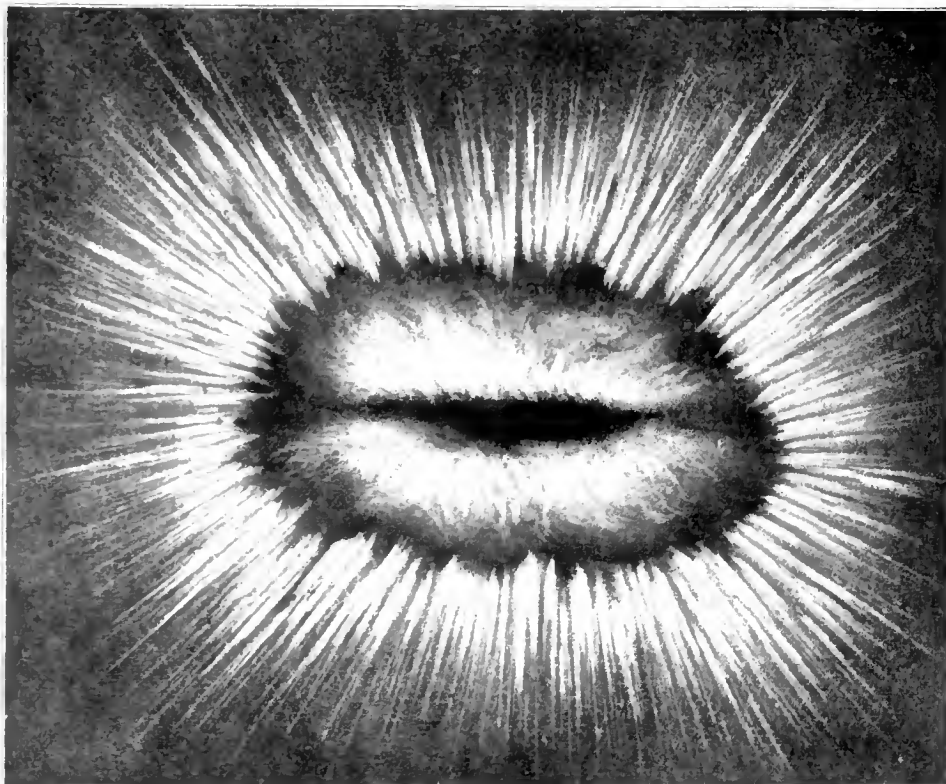
FIG. 5.—AURORAL CORONA.
